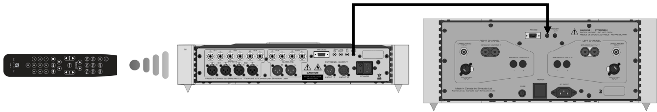
Figure 5: Commande à distance à déclencheur de 12 volts
