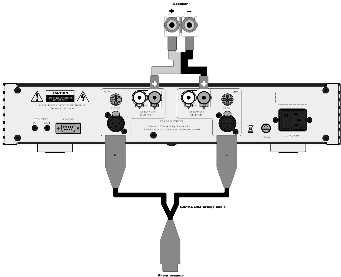
Figure 3: Utilisation en mode Mono du Nêo 330A
